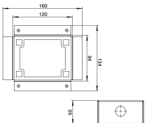
Caixa pré-instalação Pre-installation box Caja de preinstalación Boîte de pré-installation
