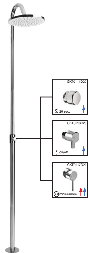
Coluna duche inox chuveiro Ø20cm S. Steel shower column Ø20cm Columna ducha inox rociador Ø20cm Colonne douche inox pomme Ø20cm
